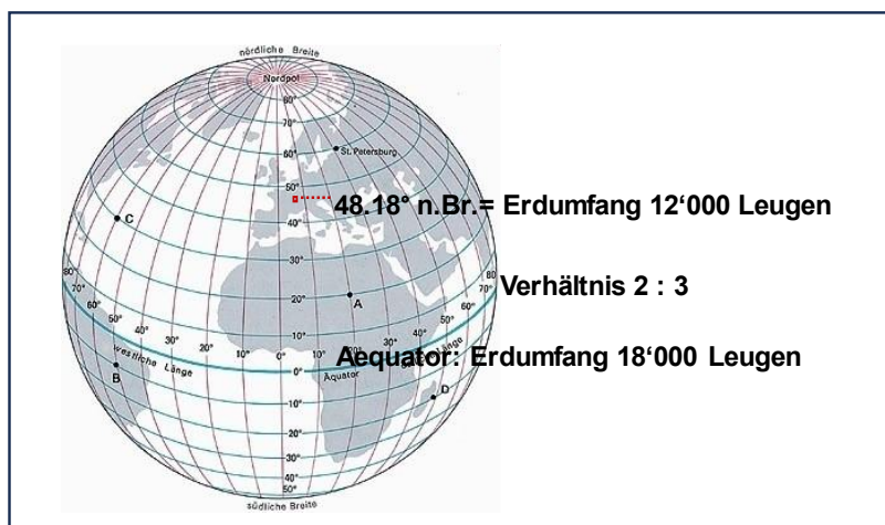
Abbildung 8: Erdkugel mit \frac{2}{3} Erdumfang bei 48.18^\circ .
