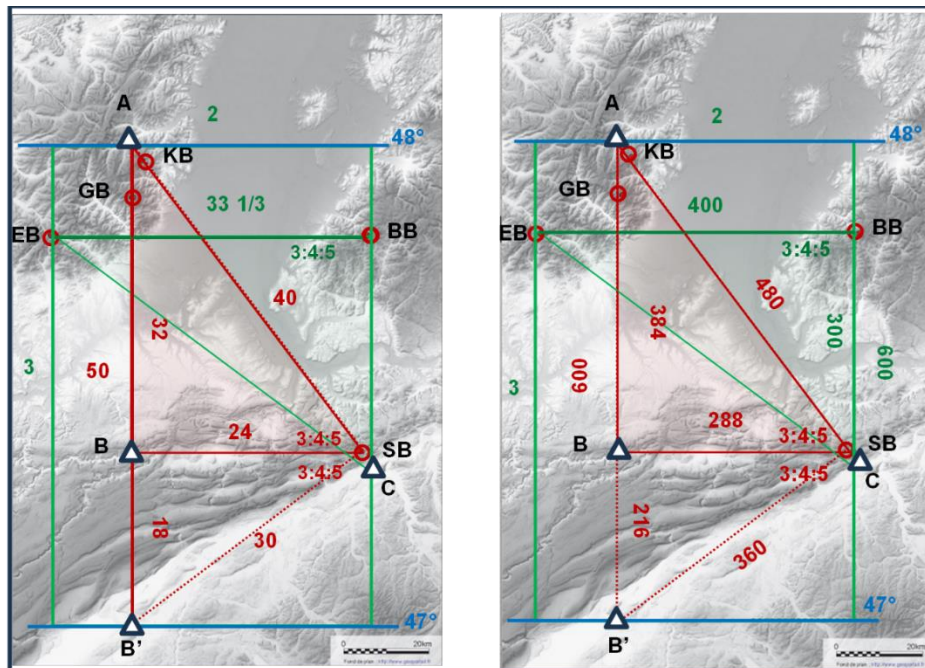
Abbildung 9: Geometrie und Masse der geodätischen Bogengradeinheit. Masszahlen links in Leugen (2221,4 m), Masszahlen rechts in Stadien (185,12 m).
